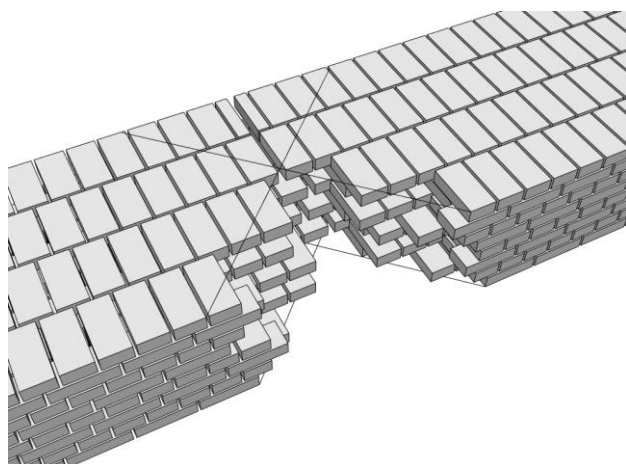
Afbeelding 6: Voorbereiding herstel transversaalscheur
